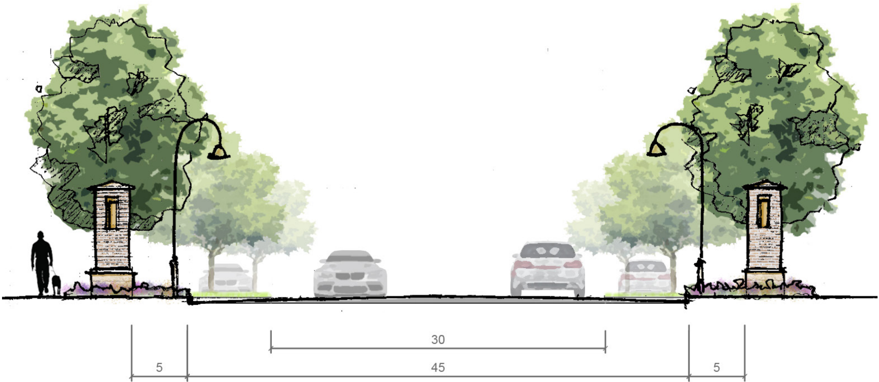
SECTION A-A
